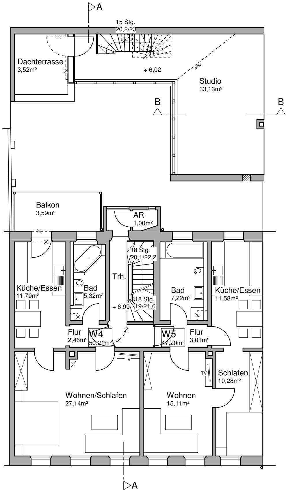
2. Obergeschoss
